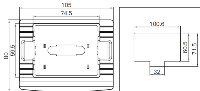
Основные и монтажные размеры панели управления (единица измерения: мм)
