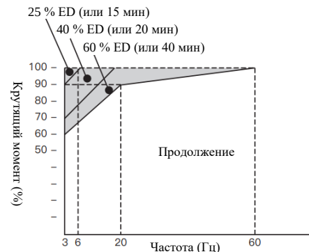
Допускаемые характеристики нагрузок стандартных двигателей
